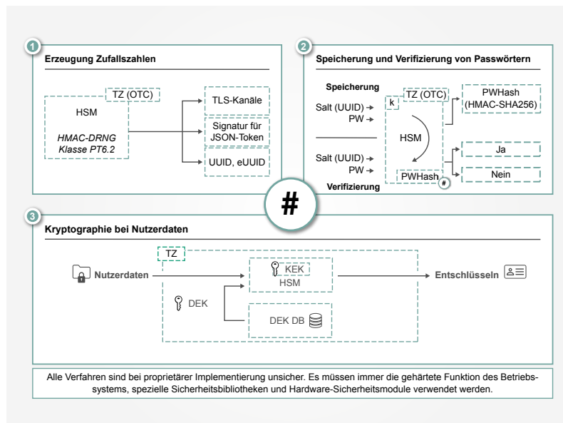
Abbildung 3: Überblick Methoden für Generierung kryptographischer Schlüssel
