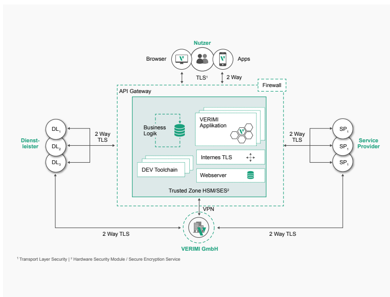
Abbildung 2: Überblick Sicherheitsarchitektur VERIMI
